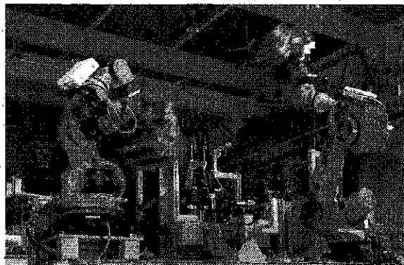
アルミダイカストロボットシステム
